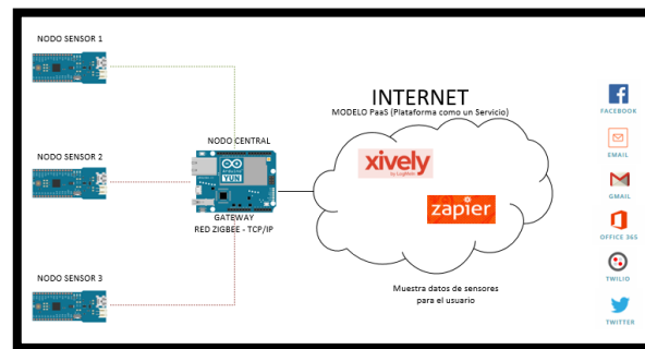
Fig. 5 Esquema de Sistema de monitoreo
