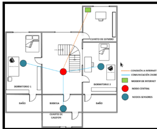
Fig. 11 Ubicación nodos sensores y central
