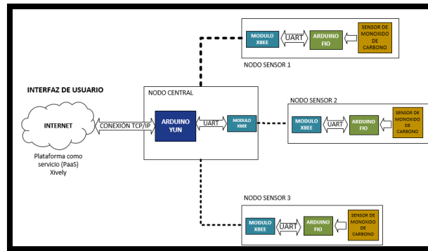
Fig. 4 Arquitectura del Sistema
