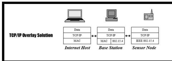
Fig. 3 Solución mediante Overlay
